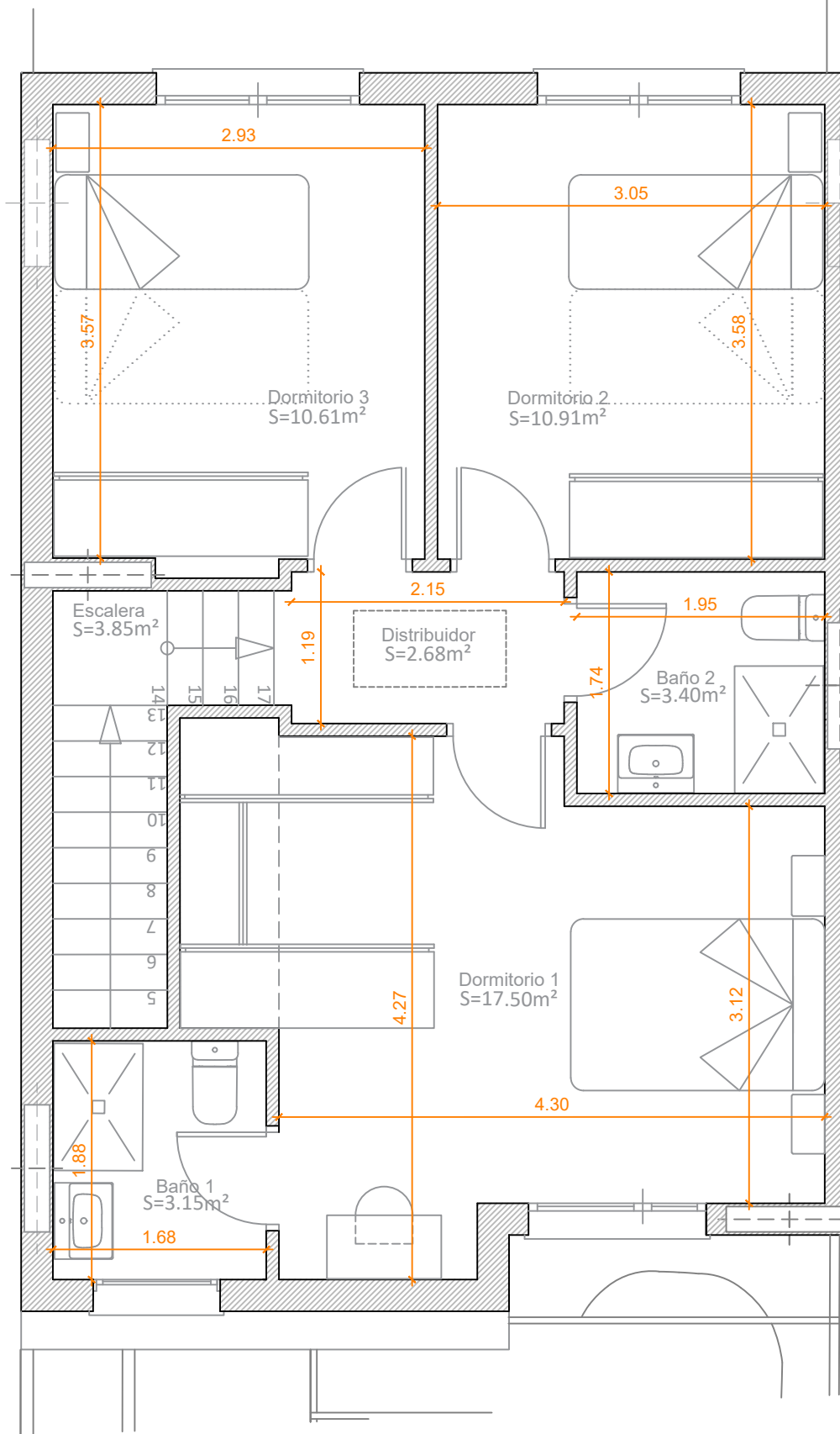
Planta Alta S=48,25m 2
