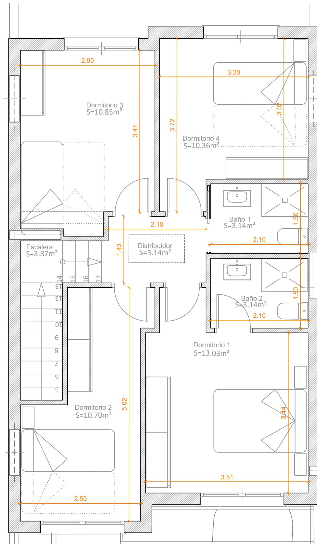
Planta Alta S=54,36m 2
